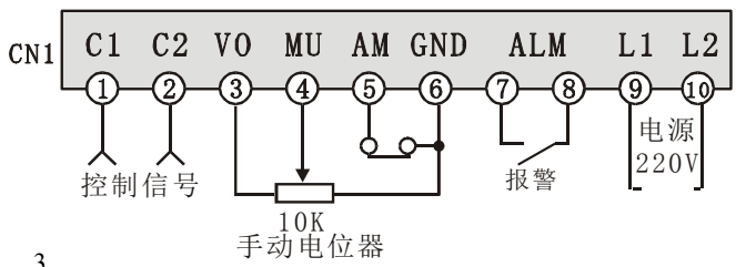
图3: 自动+手动控制接线图。
